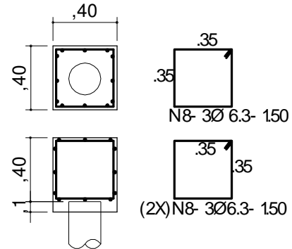
FORMA E ARMAÇÃO DOS BLOCOS DE FUNDAÇÃO (15)
