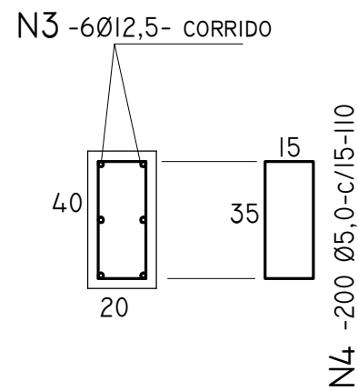
VIGA INFERIOR- 20X40
