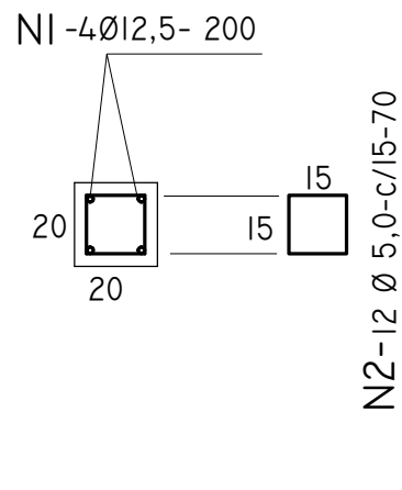
PILARES- 20X20 (15X)
