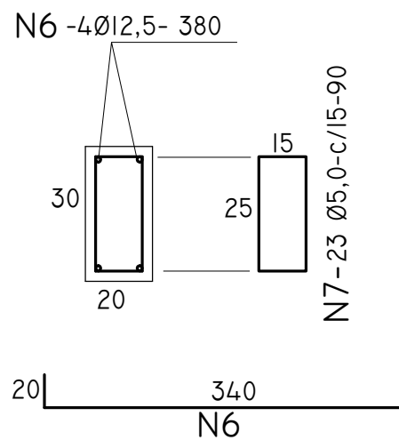
TIRANTES- 20X30 (15X)
