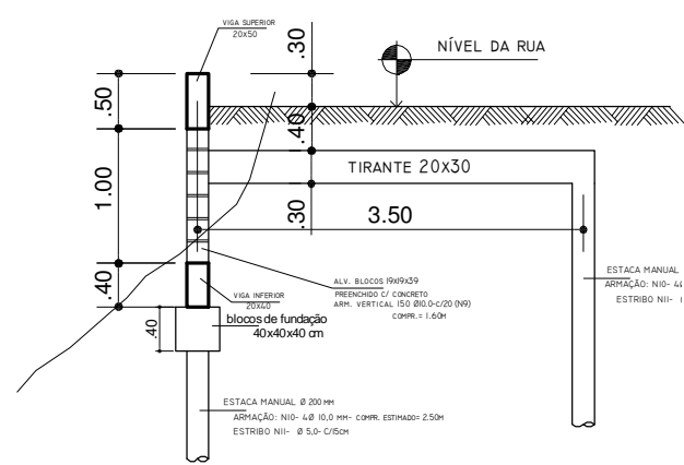
SEÇÃO A-A (GENÉRICA)
