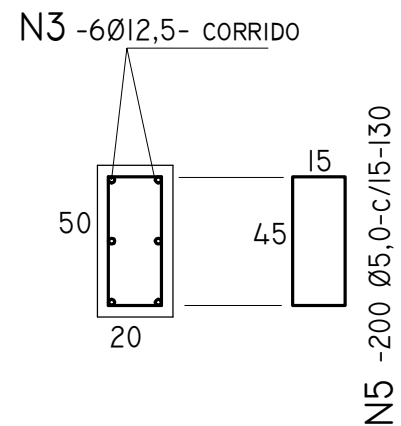
VIGA SUPERIOR- 20X50
